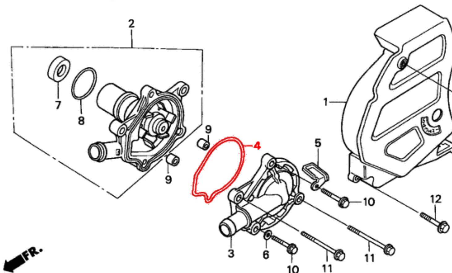
Schemat: Honda XL600V Transalp
